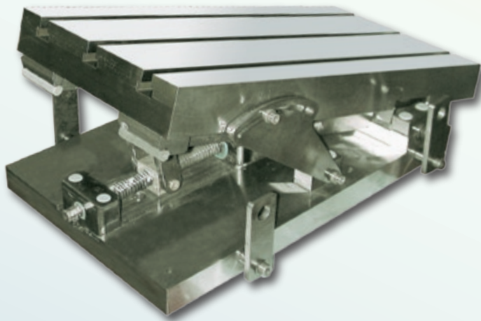
Präzisions-Sinus-Messtisch Precision measuring sine table
